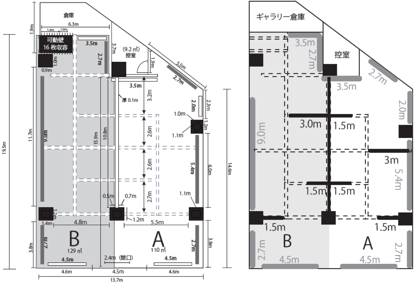
ギャラリー図面(実測値記入版)
